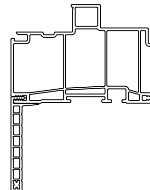
2" FLUSH FIN
